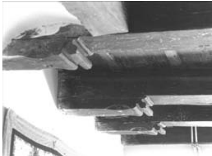
Het Houten Huys op het Begijnhof aan het begin van de twintigste eeuw en enkele sleutelstukken in het souterrain in 1994 (foto's BMA).
