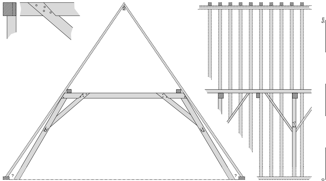
Doorsnede van de laatmiddeleeuwse kap van Barndesteeg 4-6 (tekening David Derksen, BMA).
