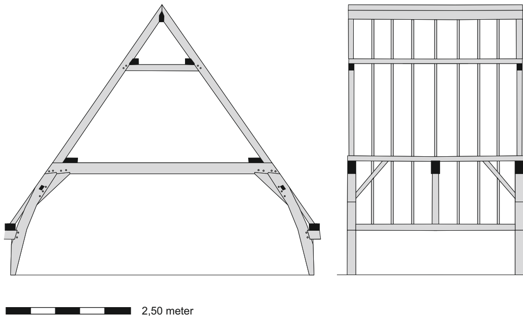
Nieuwezijds Voorburgwal 284, kapconstructie (tekening auteur/ BMA).
