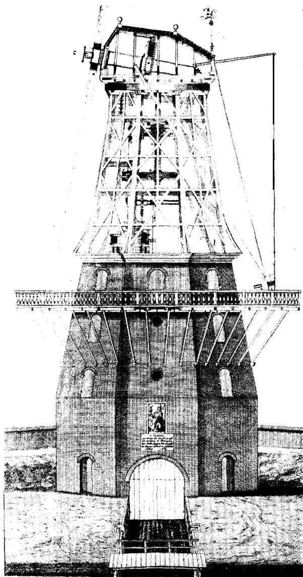
De korenmolen Sint Victor. Bouwkundige teekening uit het Molenboek van Pieter Limpergh, moolenmaker van Stockholm, nieuylks in plaatdruk uytgegeeven door Justus Danckerts. ± 1700. (Verzam. G. J. Honig).
